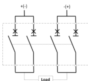
2P 产品 4P 外形接线图(DC440V)
