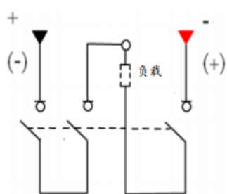
3P外形接线图(DC750V)
