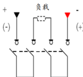
4P外形接线图(DC1000V)
